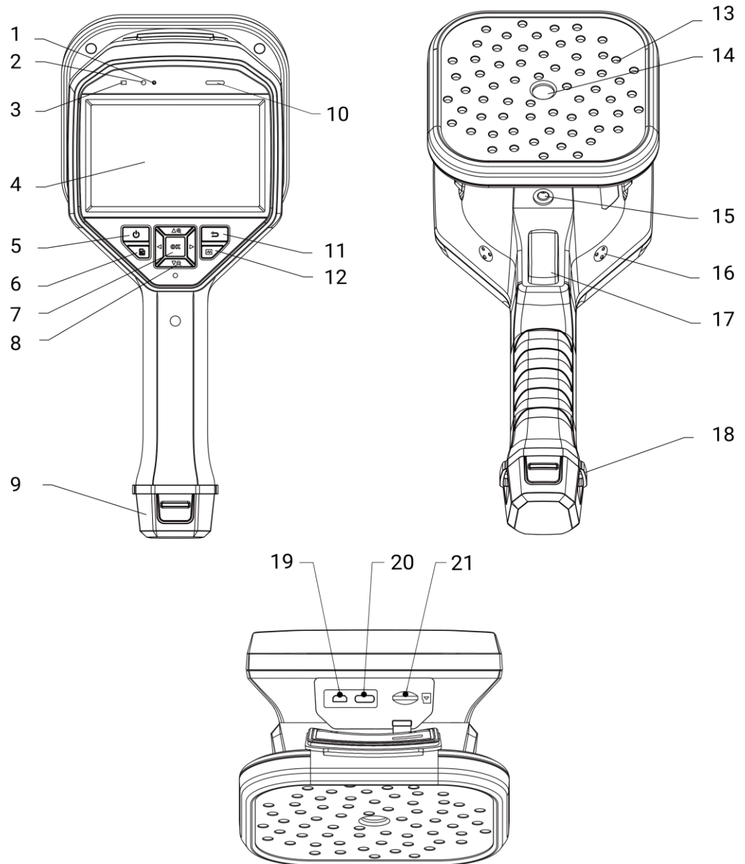
그림 1-1 외관: 64-마이크 어레이
