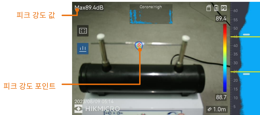
그림 5-2 피크 강도 마킹
