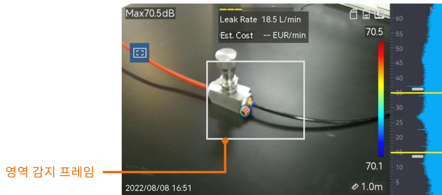
그림 5-3 영역 감지 프레임
