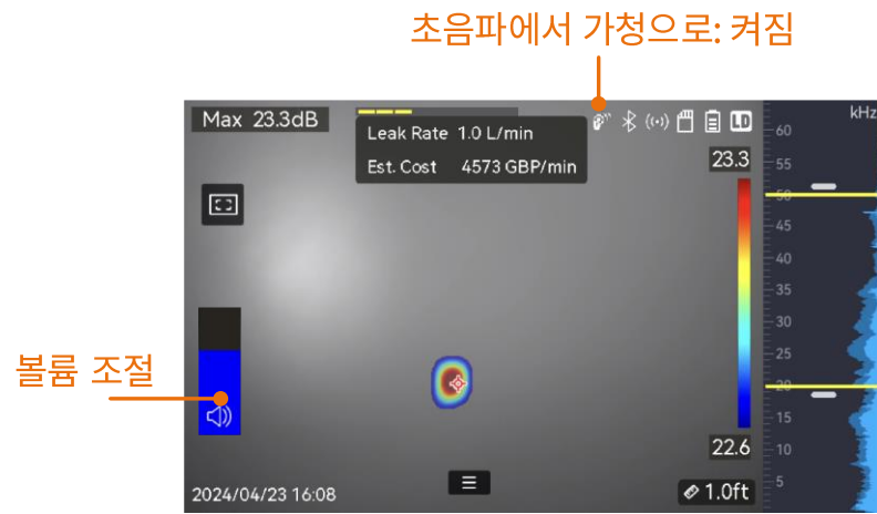
그림 5-4 '초음파에서 가청으로' 및 볼륨 조정
