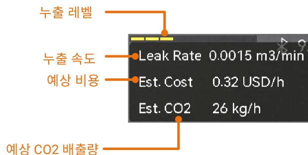
그림 4-2 가스 누출 추정(압축 공기)
