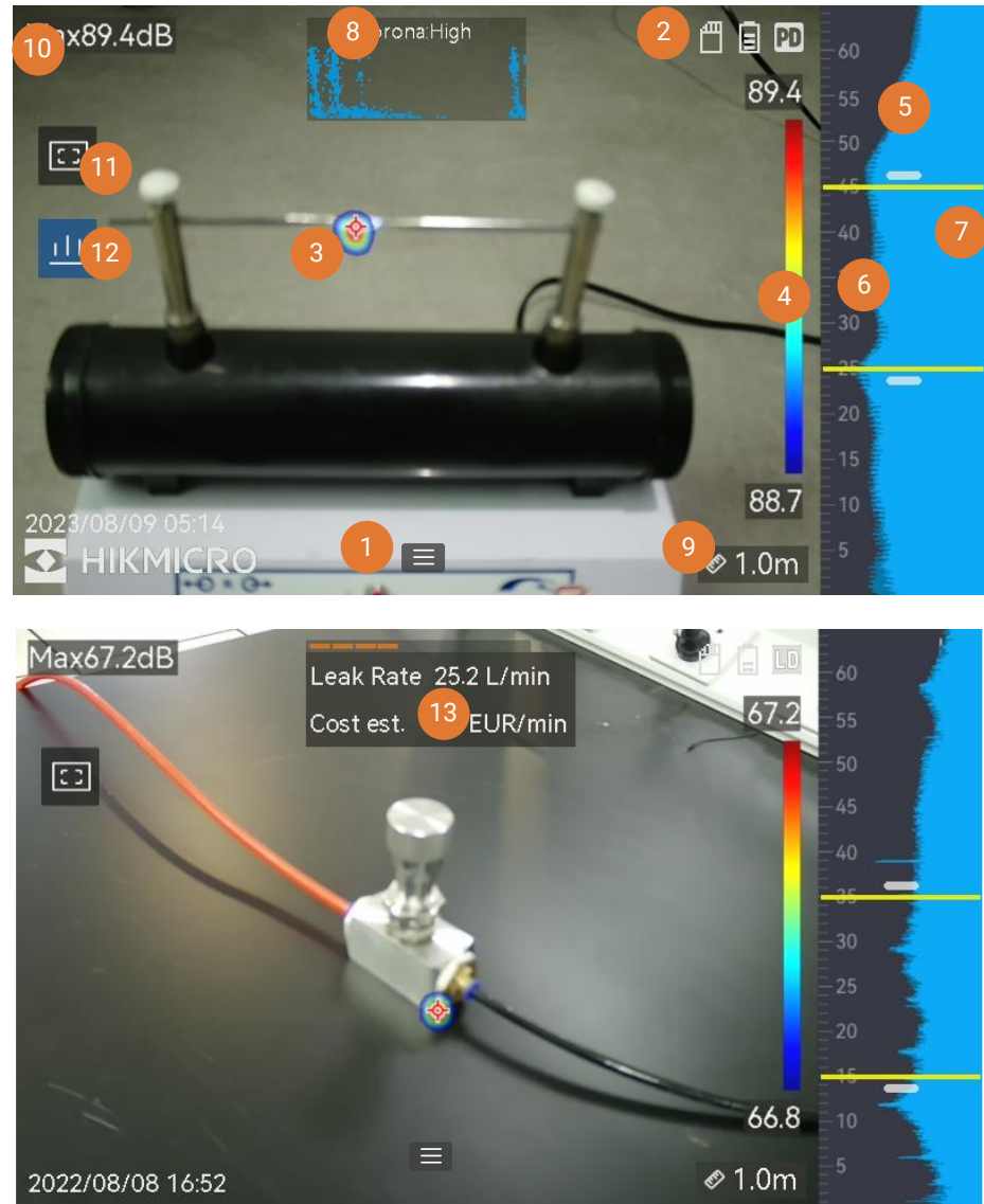
그림 2-8 실시간 보기 인터페이스
